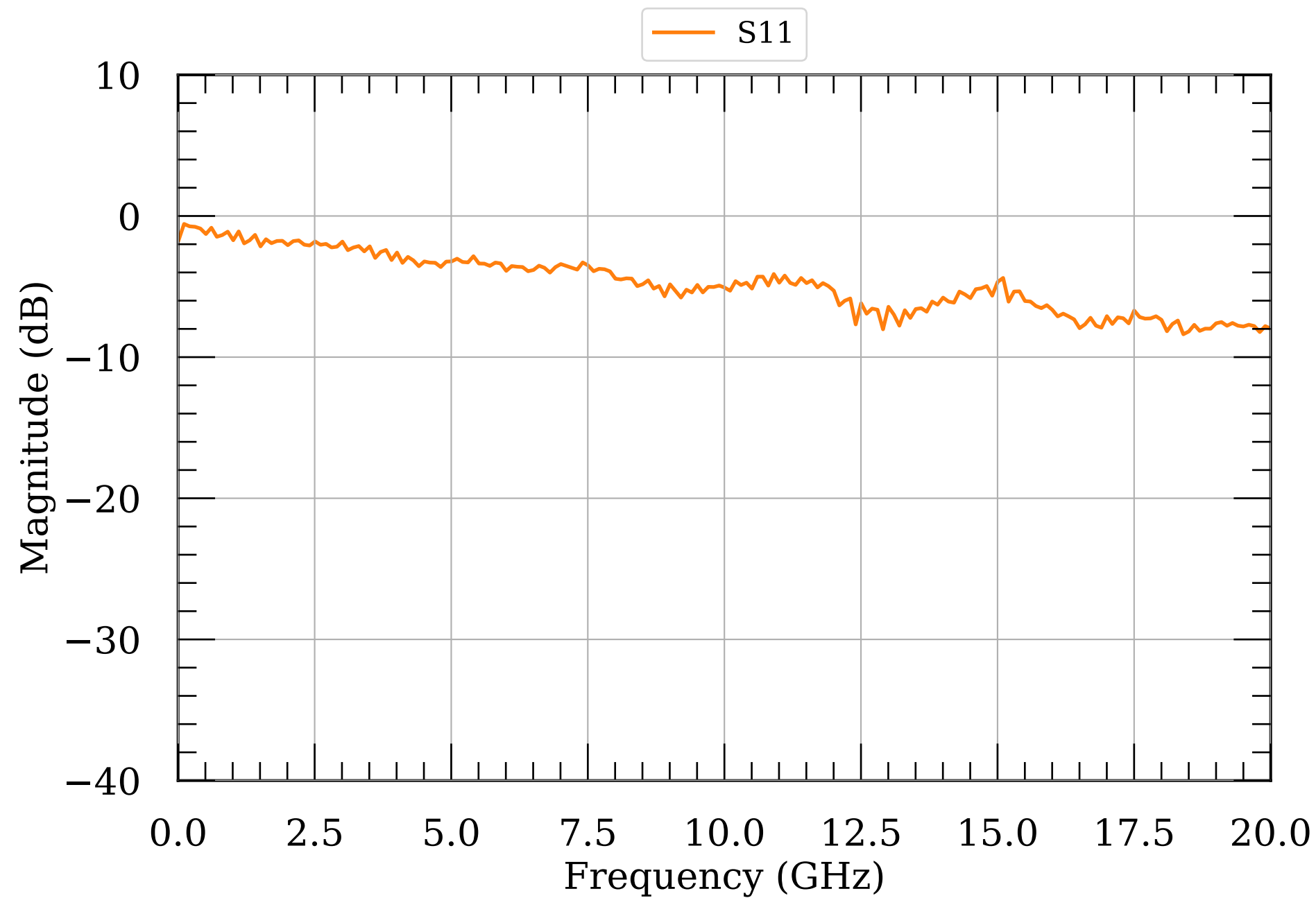
LNA S-params module078
